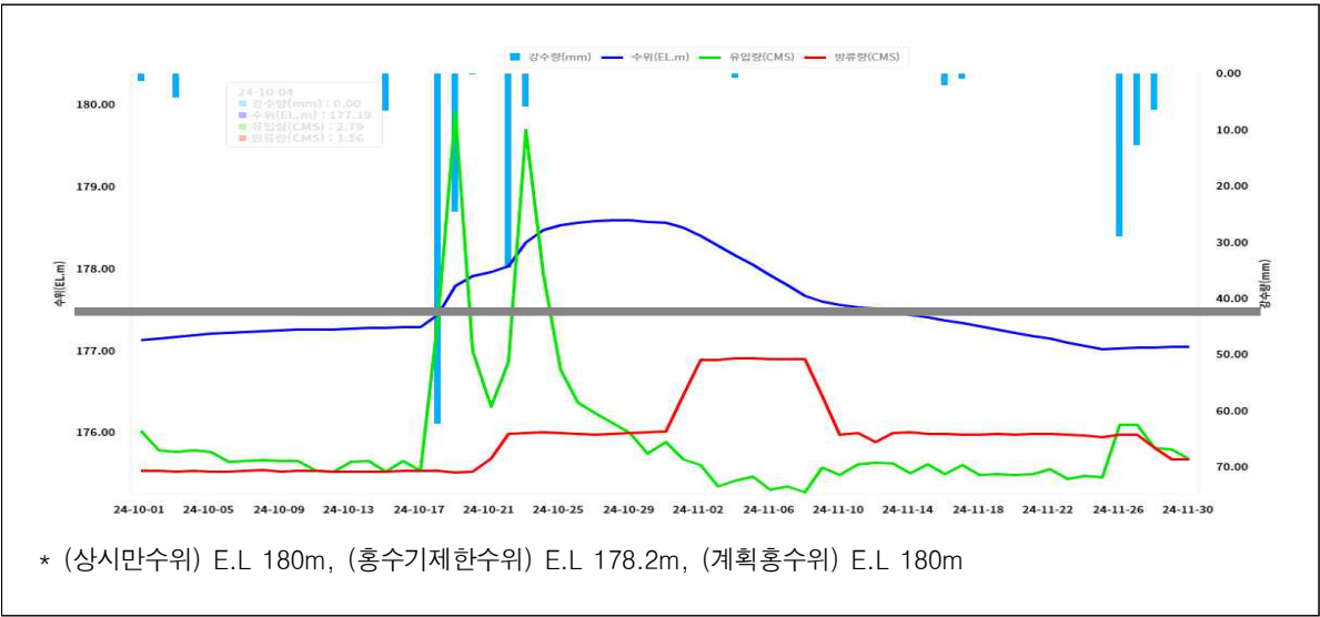
[그림 2] 댐 호수길(E.L 177.6m) 침수에 따른 수위조절 현황(2024년)
